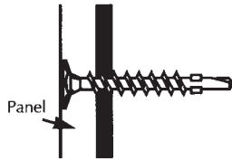
Fig. 3 Metal Stud
